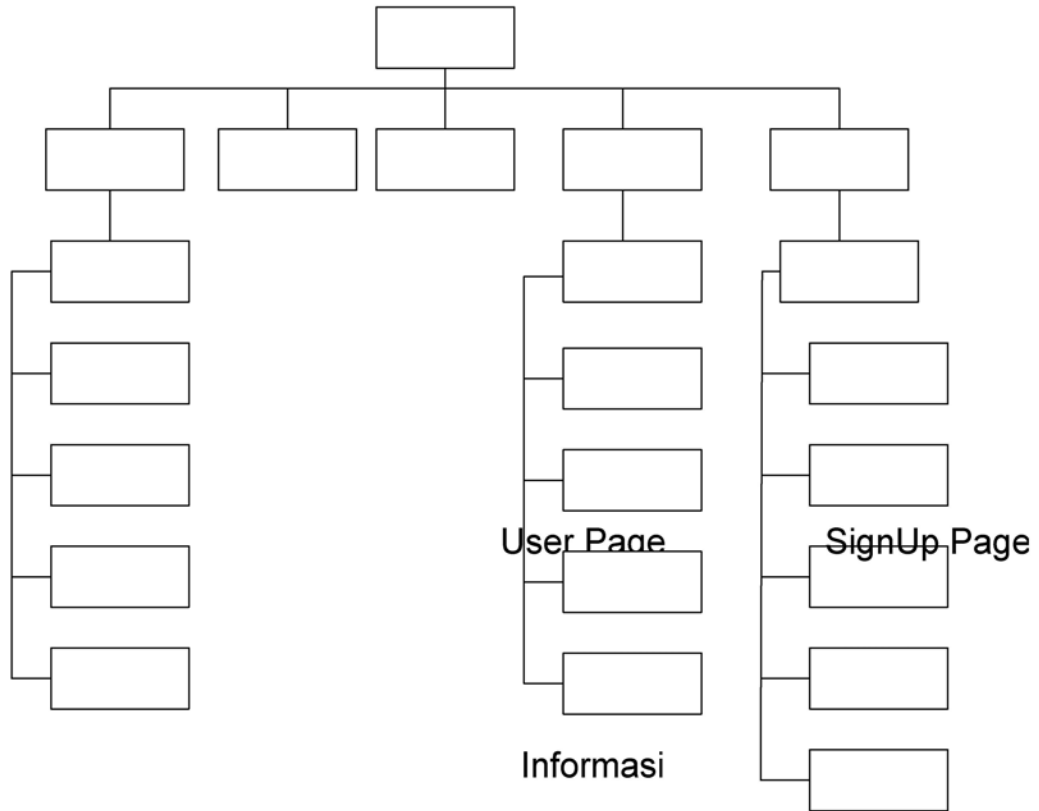
Gambar 5.4 Struktur Program
