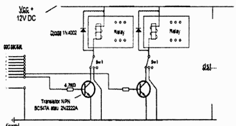
Gambar 4. Diagram Rangkaian Perangkat Antarmuka
