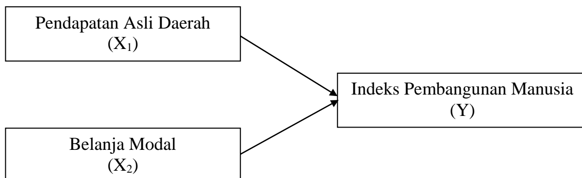
Gambar 1. Hubungan Struktur X 1 , X 2 terhadap Y
